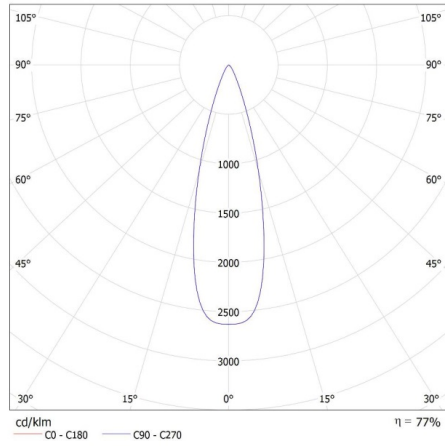
KANLUX S.A. (kat 35650) BTL 18W-930-W 15deg + GRID / LDC (Polar)
