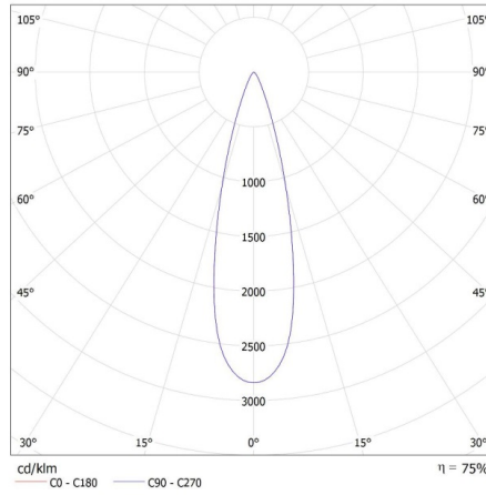
KANLUX S.A. (kat 35651) BTL 18W-930-B 15deg + GRID / LDC (Polar)
