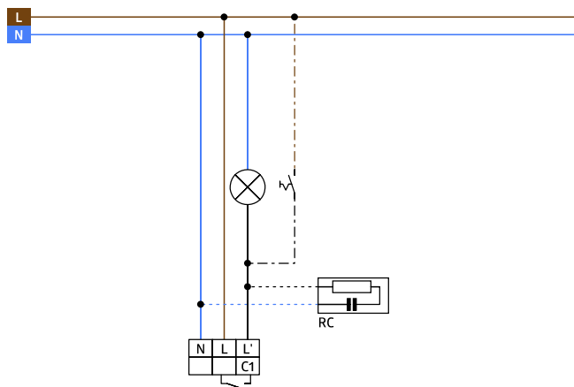
Kapcsolási rajzok
